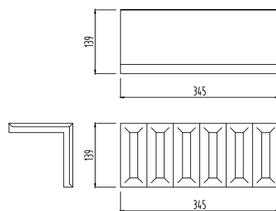
základní kachel přímý 14 x 35 4,9 jednotek
