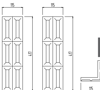
roh ostrý zmenšený 42 x 11,5 4,9 jednotek
